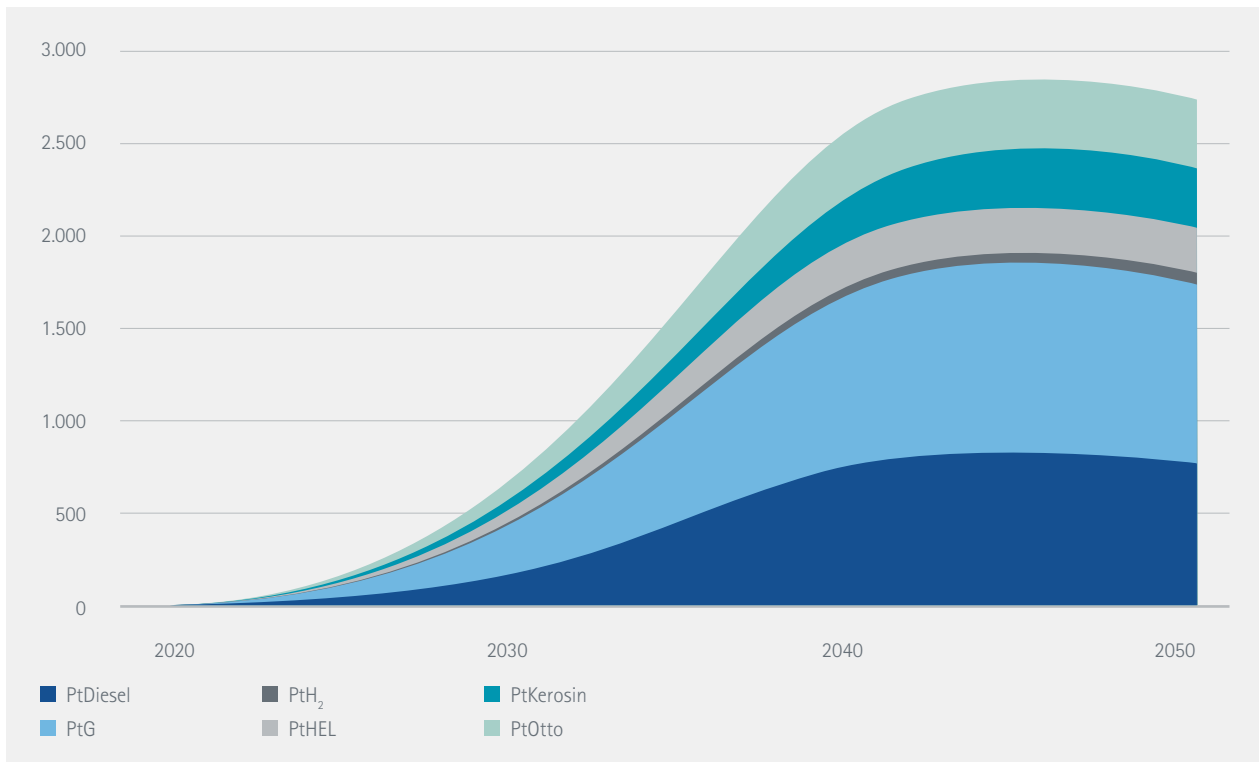
Abbildung 33: Szenario PtX 80 – Einsatz synthetischer Energieträger 2020 – 2050, in PJ
